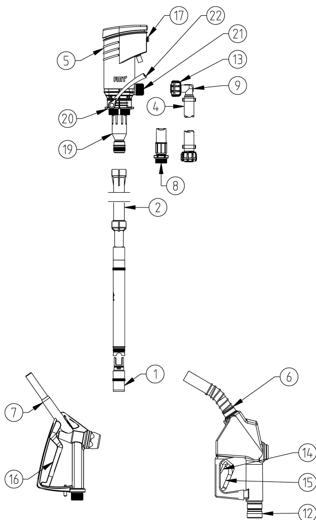
Obr: 6-1: Přehled PREMAxx Diesel s příslušenstvím
