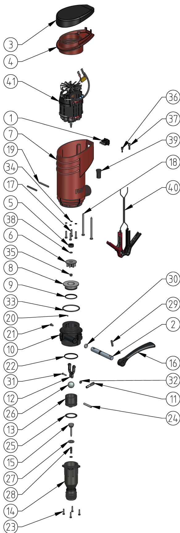
Obr: 14 - 1: Rozložený pohled PREMAxx dieselové čerpadlo 24/12 V
