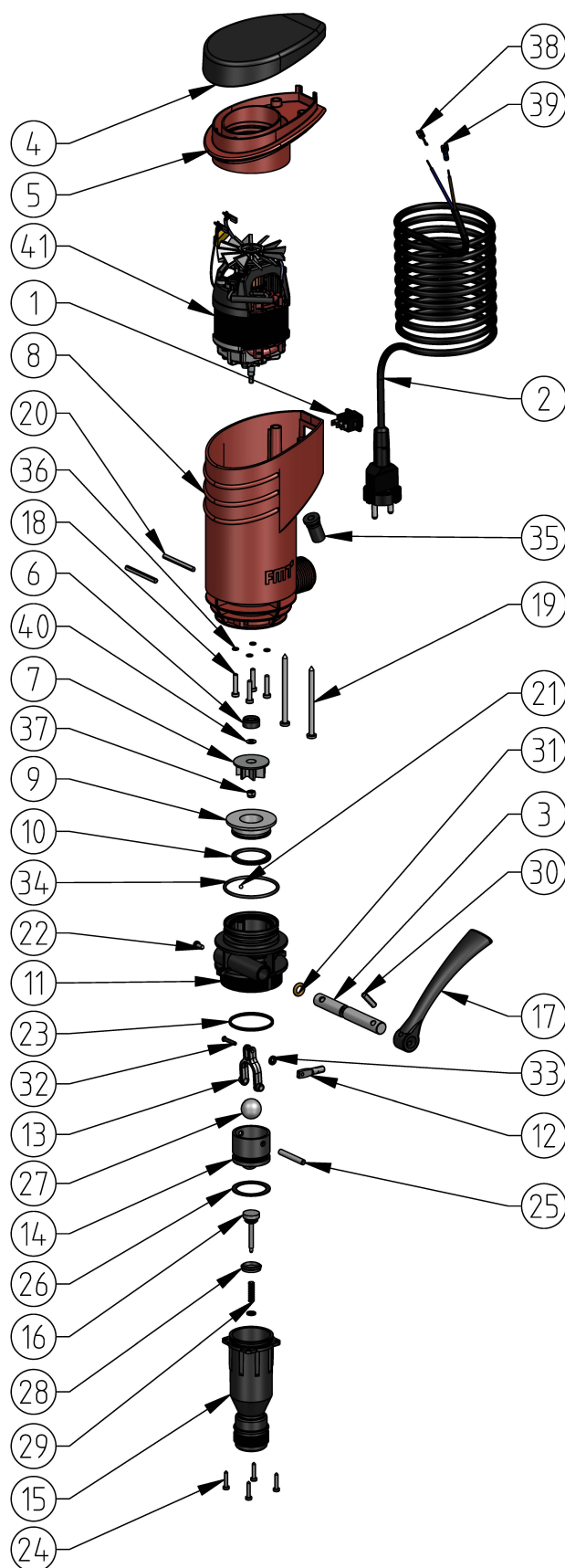
Obr: 13 - 1: Rozložený pohled PREMAxx dieselové čerpadlo 230 V
